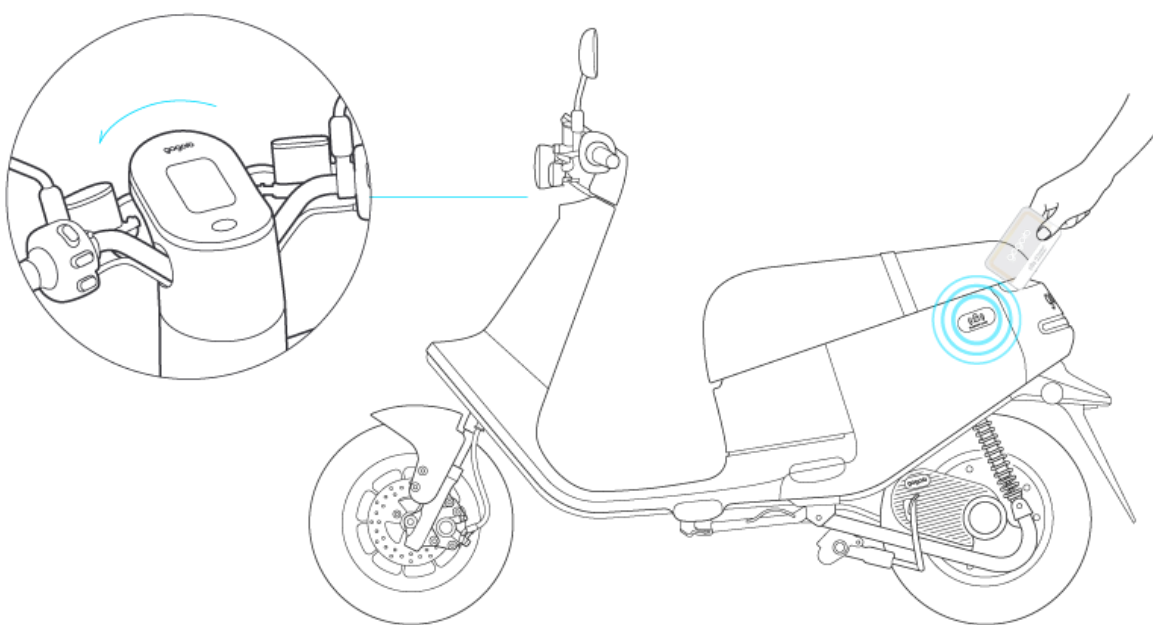
iQ System® 智慧鑰匙卡感應器位置
